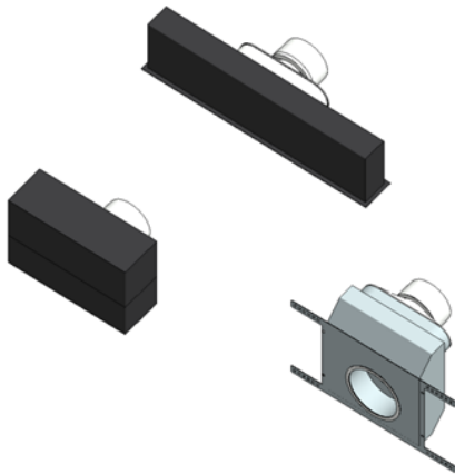
Luchtverdeelboxen zonder roosters en kleppen
